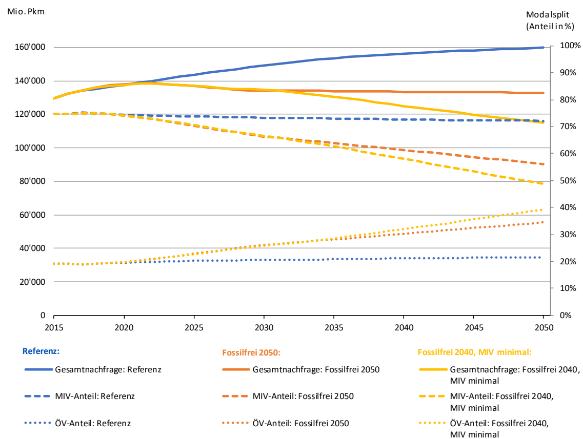
Abbildung 41: Entwicklung Verkehrsleistung (pkm) und Modalsplit im Personenverkehr je Szenario
